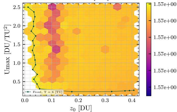
Period = 6 [TU]
