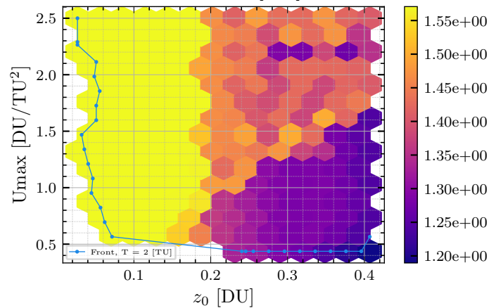
Period = 2 [TU]
